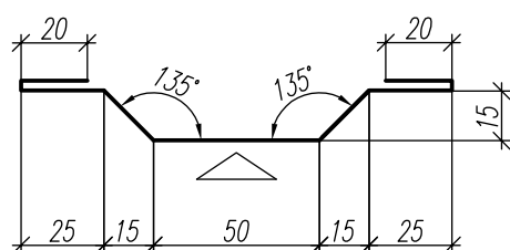
ФЭ-С2 (Фасонный Элемент Стеновой 2).
