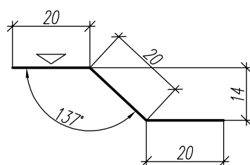
ФЭ-4 (Фасонный Элемент 4).
