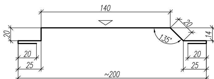
ФЭ-С4а (Фасонный Элемент Стеновой 4а).
