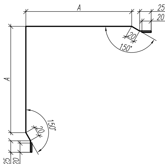
ФЗ-У1 (Фасонный Элемент Угловой 1)
