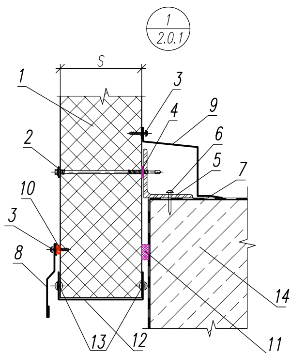
ФЭ-Ц1 (Фасонный Элемент Цокольный 1)
