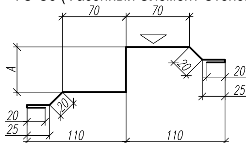
ФЭ-С8 (Фасонный Элемент Стеновой 8).
