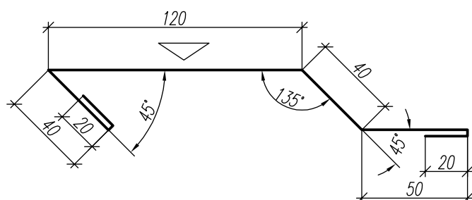
ФЭ-О1 (Фасонный Элемент Оконный 1)
