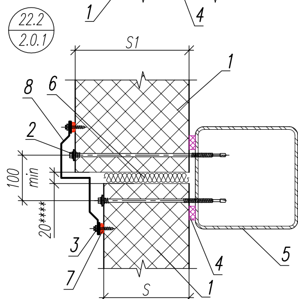
ФЭ-С8 (Фасонный Элемент Стеновой 8).
