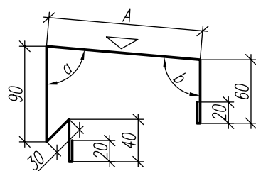
ФЭ-НК16 (Фасонный Элемент Кровельный 16).
