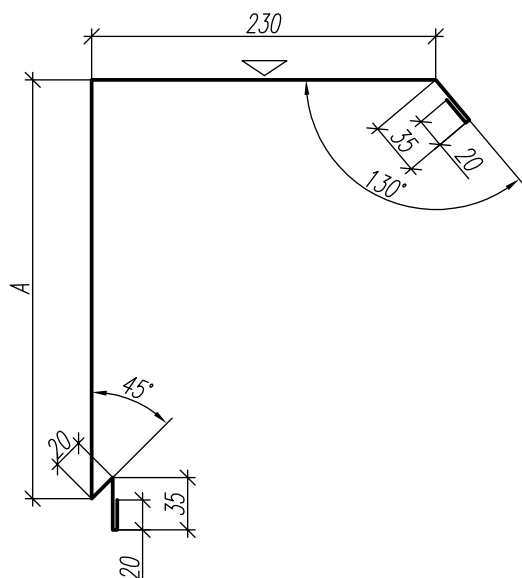
ФЭ-НК11 (Фасонный Элемент Кровельный 11).
