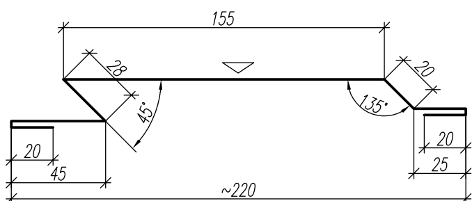
ФЭ-4 (Фасонный Элемент 4).
