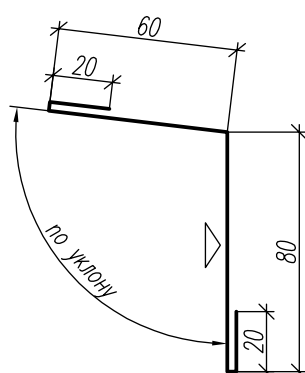
ФЭ-НК2(Фасонный Элемент Кровельный 2).
