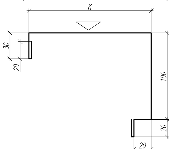
Геометрические х-ки ФЭ-В1
