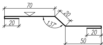
ФЭ-Ц2 (Фасонный Элемент Цокольный 2)
