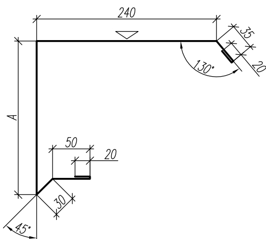
ФЭ-НК13 (Фасонный Элемент Кровельный 13).
