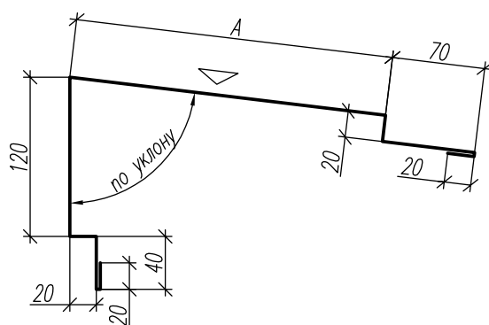
ФЭ-НК3(Фасонный Элемент Кровельный 3).
