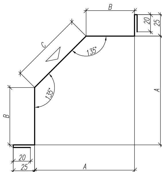
ФЭ-С3 (Фасонный Элемент Стеновой 3).
