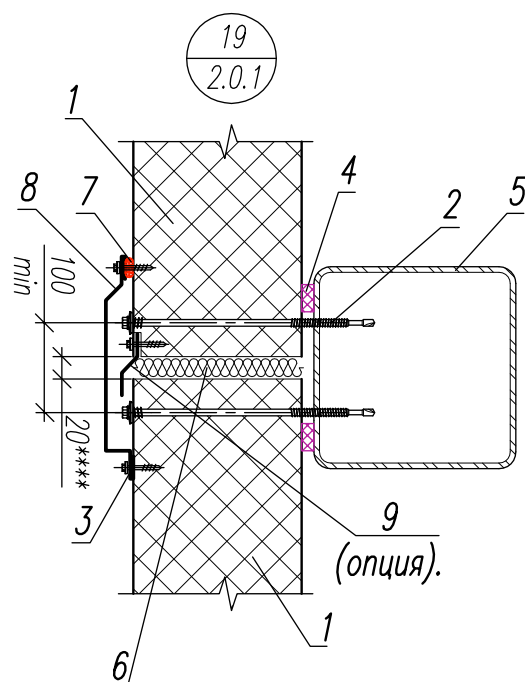
ФЭ-С4 (Фасонный Элемент Стеновой 4).
