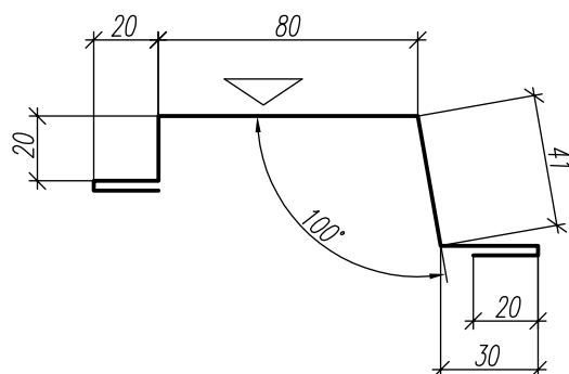
ФЭ-О3 (Фасонный Элемент Оконный 3)
