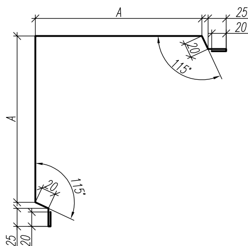
ФЗ-У1/а (Фасонный Элемент Угловой 1/а)
