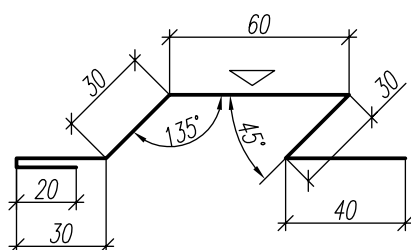
ФЭ-НК15 (Фасонный Элемент Кровельный 15).
