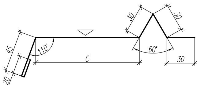
ФЭ-Ц4 (Фасонный Элемент Цокольный 4)
